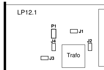
Position der Jumper ab Ver.11
