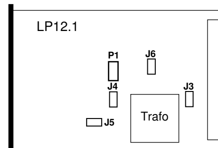
Position der Jumper bis Ver.10
